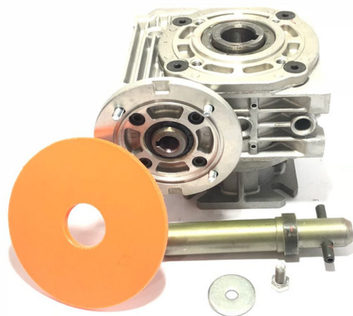
5026 - Kit redutor 3/4 CV
